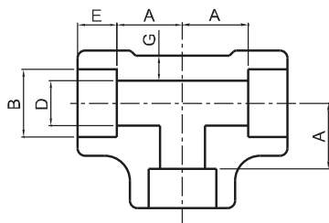
3000# (mm) ANSI B16.11
