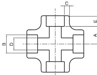
3000# (mm) ANSI B16.11
